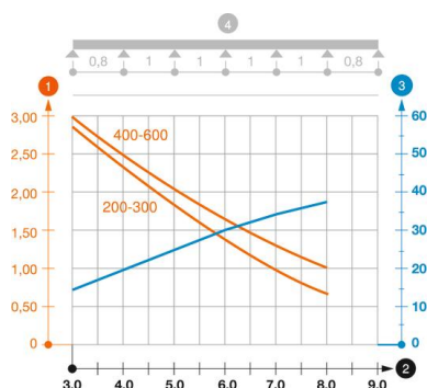
Dijagram opterećenja kabljskih polica za velike raspone tipa WKSG 160
